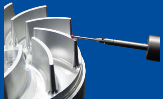
Màquina de mesura per coordenades (MMC) DEA GLOBAL PERFORMANCE 9128 equipada amb capçal TESASTAR-M i sonda de mesura en continu LEITZ LSP-X1.
